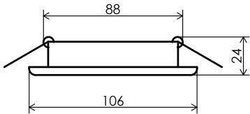
Размеры светильника
